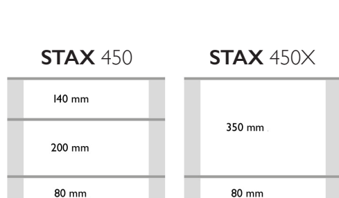
Højde: 450 mm, Bredde: 580 mm, Dybde: 400 mm
