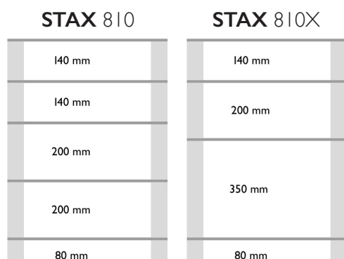
Højde: 810 mm, Bredde: 580 mm, Dybde: 400 mm
