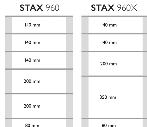
Højde: 960 mm, Bredde: 580 mm, Dybde: 400 mm
